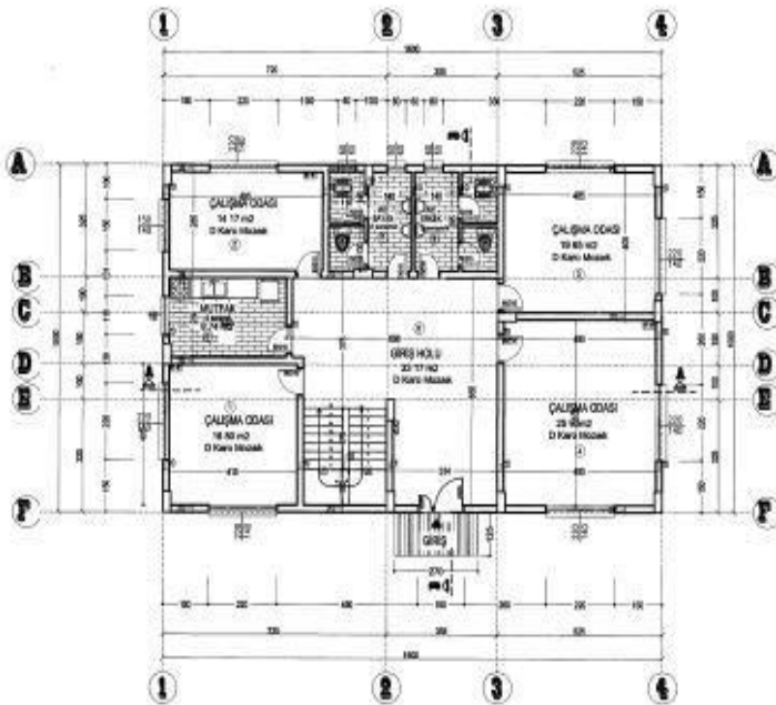
ZEMİN KAT PLANI ÖL=1/50 YATAY YÖNÜ
