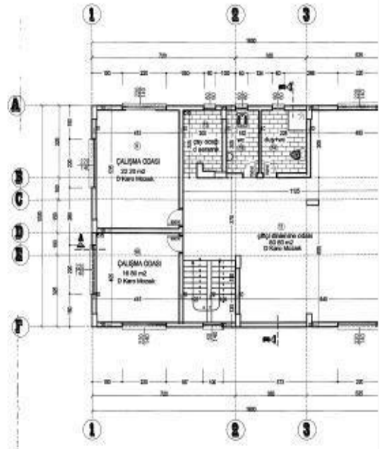
NORMAL KAT PLANI ÖL=1/50 YATAY YÖNÜ
